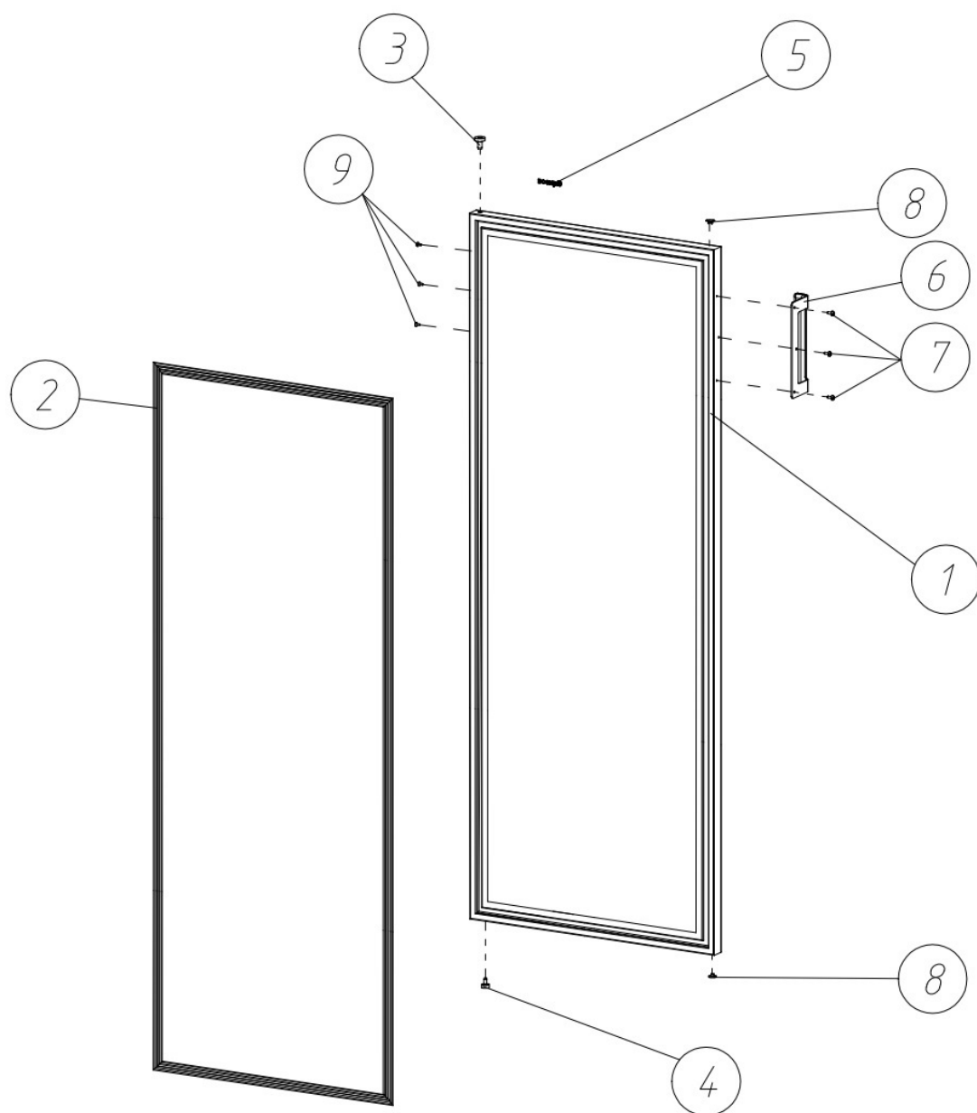
Рисунок 6 – Дверь в сборе
