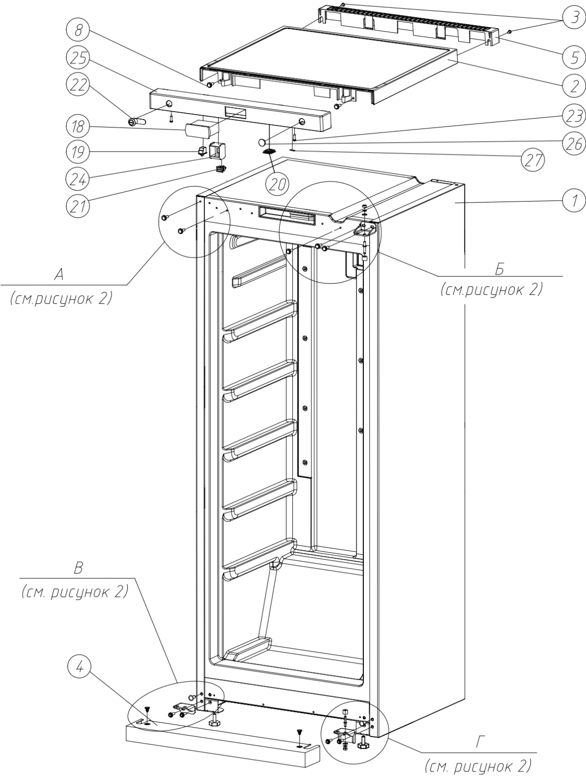
Рисунок 1 – Шкаф в сборе
