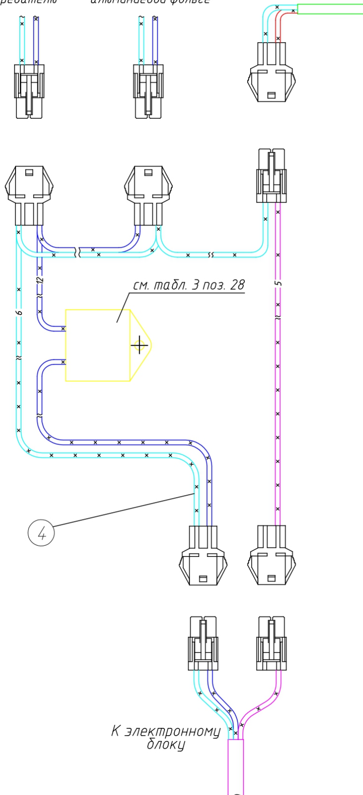
Рисунок 7а – Гирлянда сопряжения
