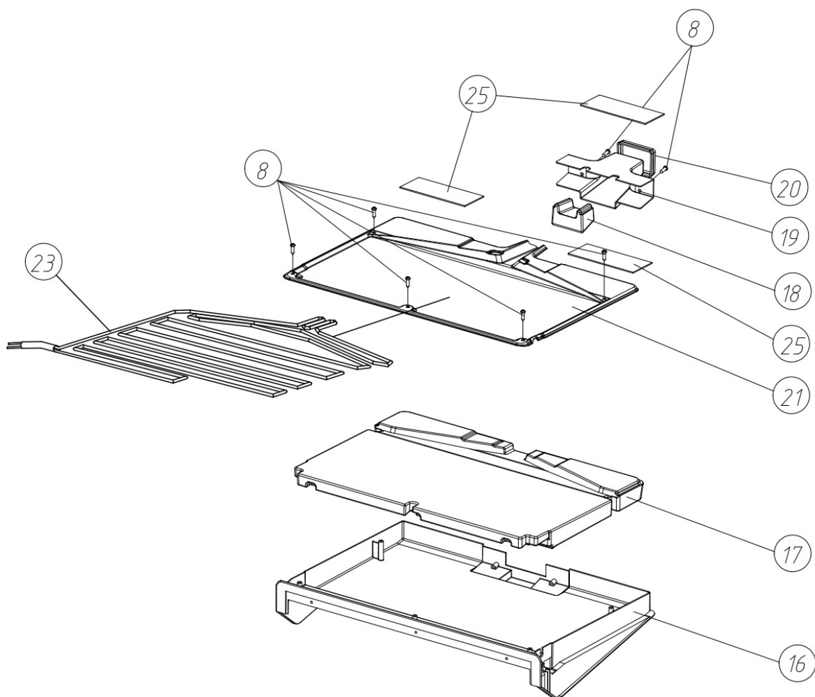
Рисунок 3б – Поддон
