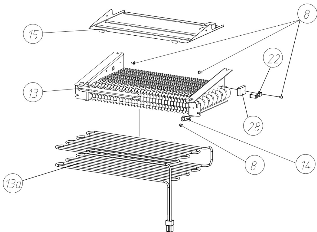
Рисунок 3а – Испаритель
