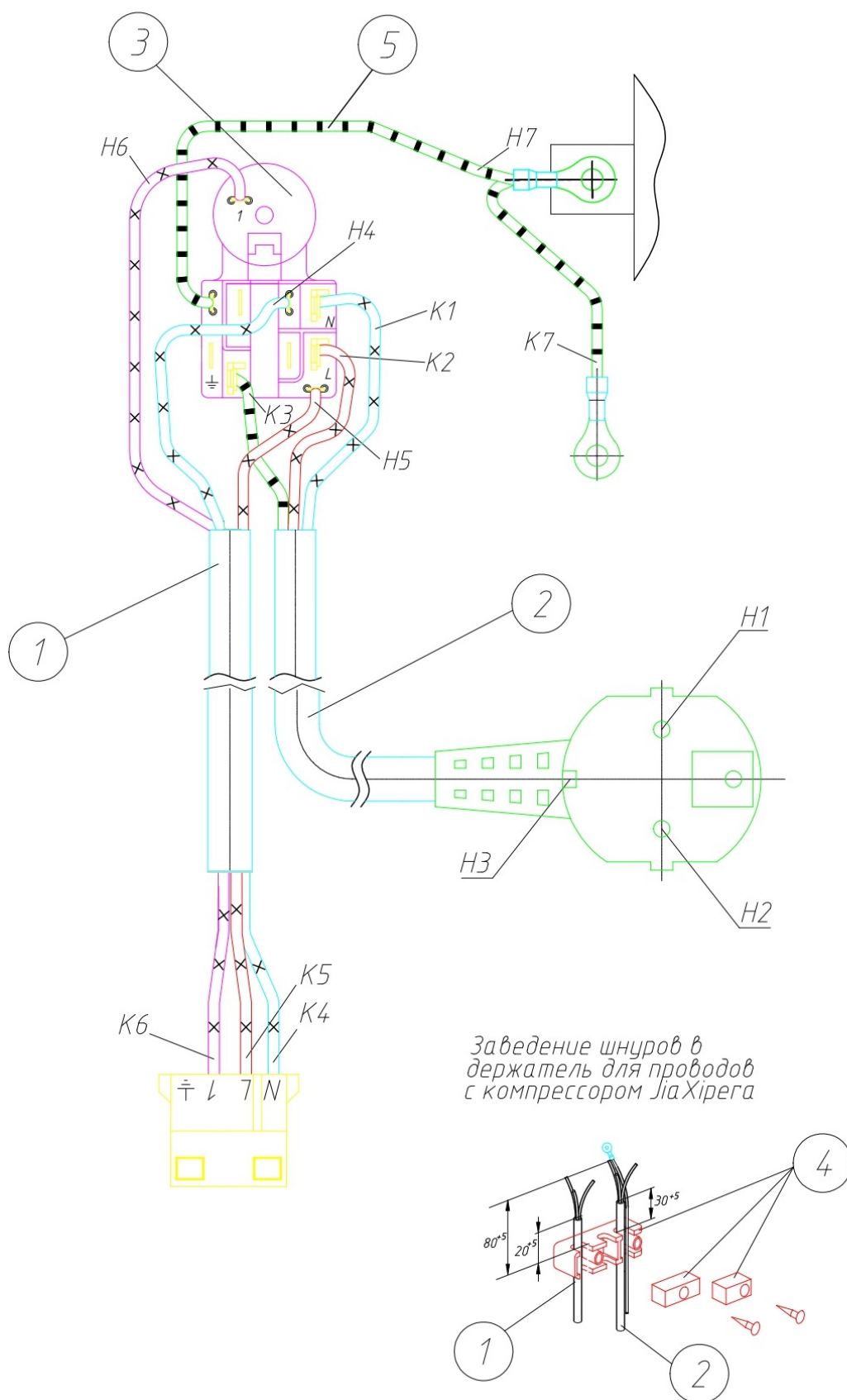
Рисунок 8 – Колодка компрессора в сборе
