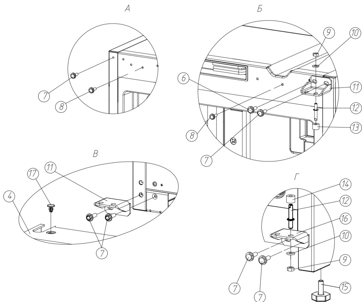
Рисунок 2 – Крепление кронштейнов
