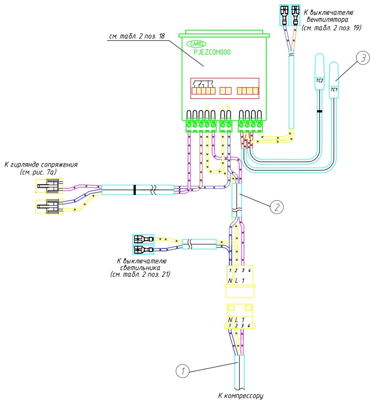
Рисунок 7 – Блок приборов
