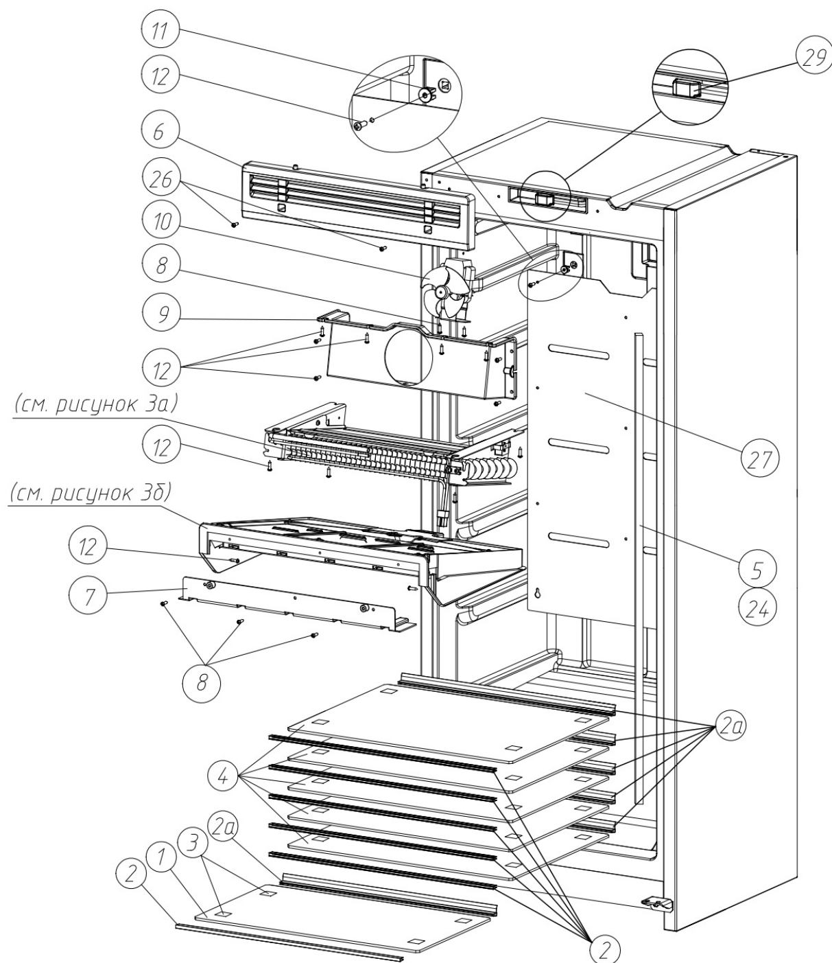
Рисунок 3 – Внутренние принадлежности
