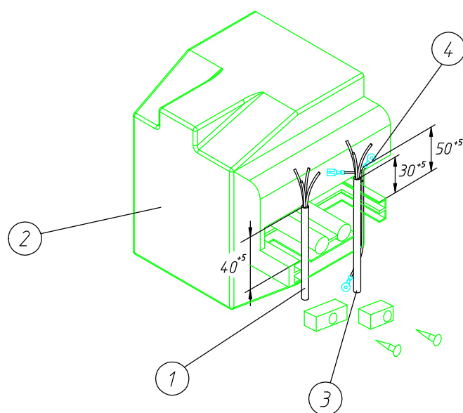
Рисунок 6а – Колодка компрессора в сборе (Daupre AG100CY1, Eateron B60CBL, GMCC SZ59C1H)
