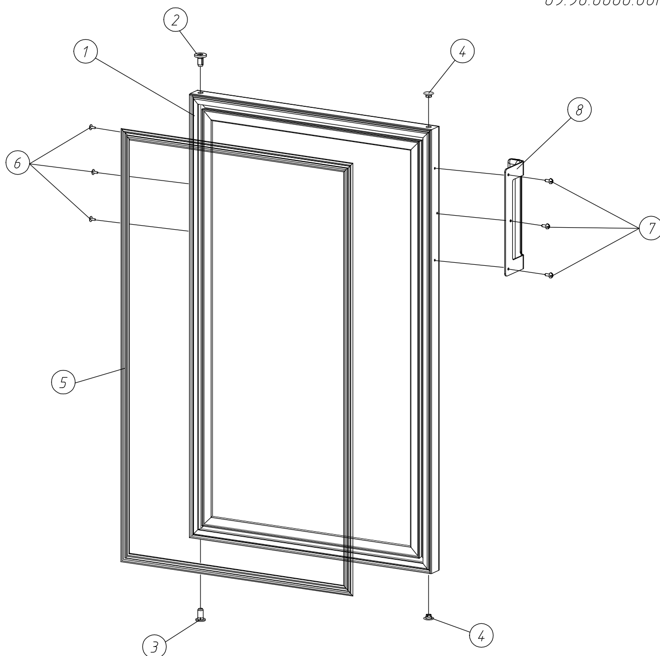
Рисунок 4 - Дверь
