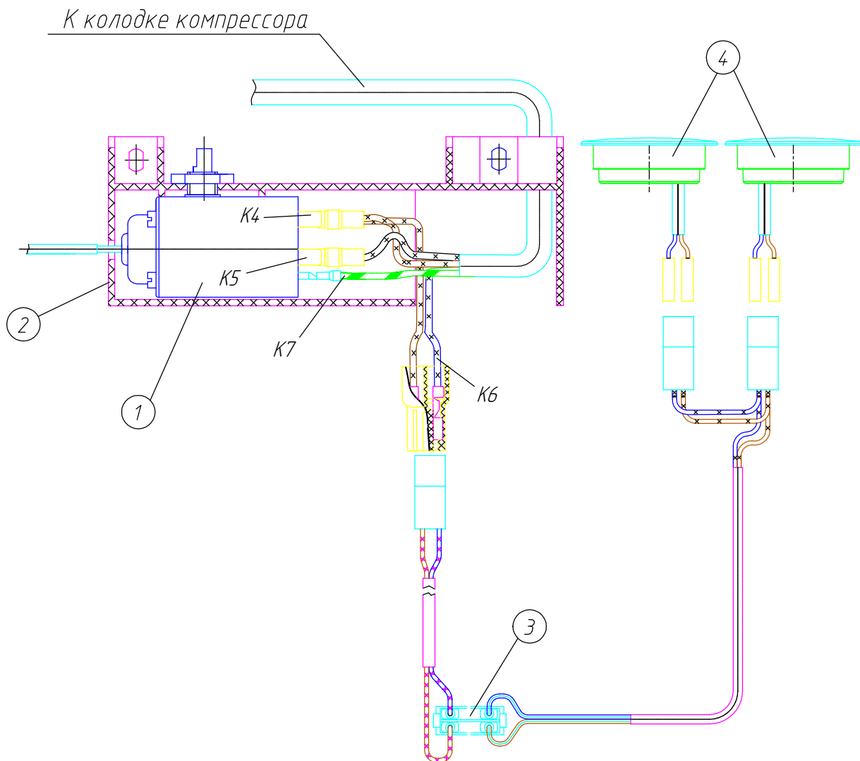
Рисунок 5а - Блок приборов (для исполнений с канале)
