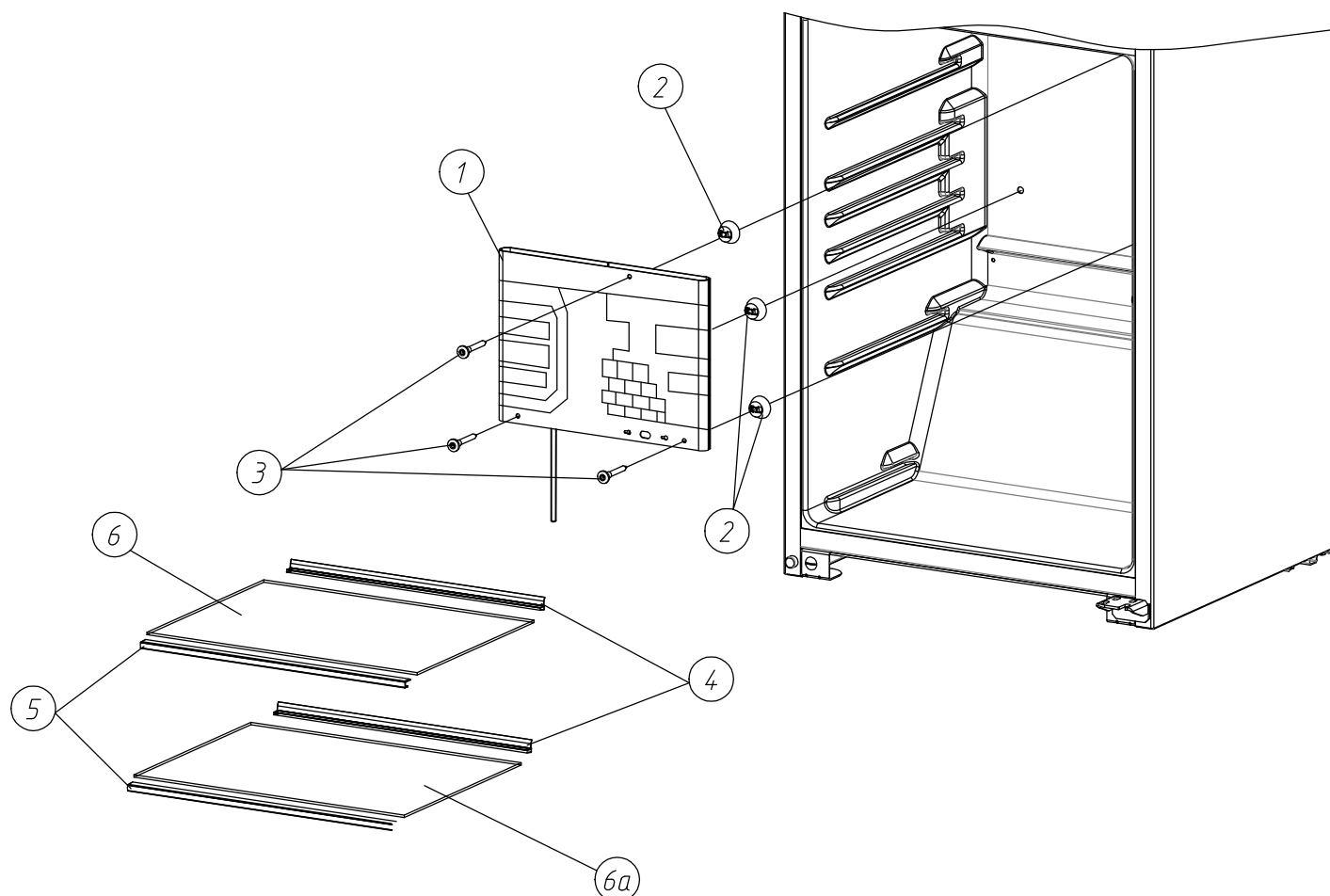
Рисунок 2 – Внутренние принадлежности
