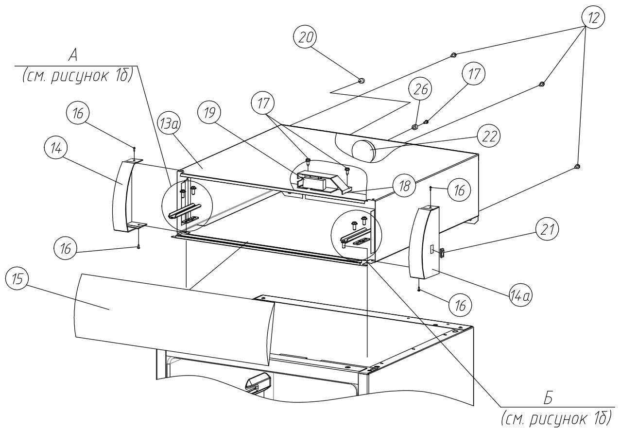
Рисунок 1а – Исполнения с канале (остальное см. рисунок 1)
