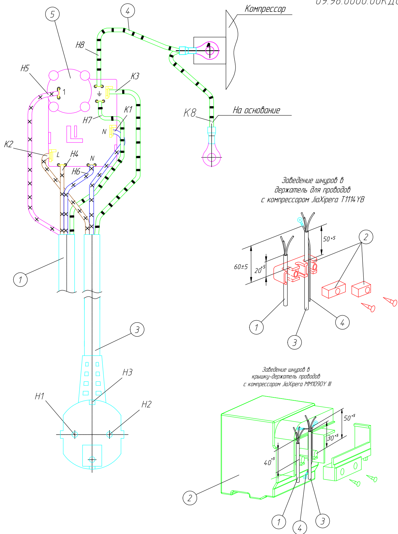
Рисунок 6 – Колодка компрессора в сборе ( JiaXipeга MM1090Y, T1114 YB)
