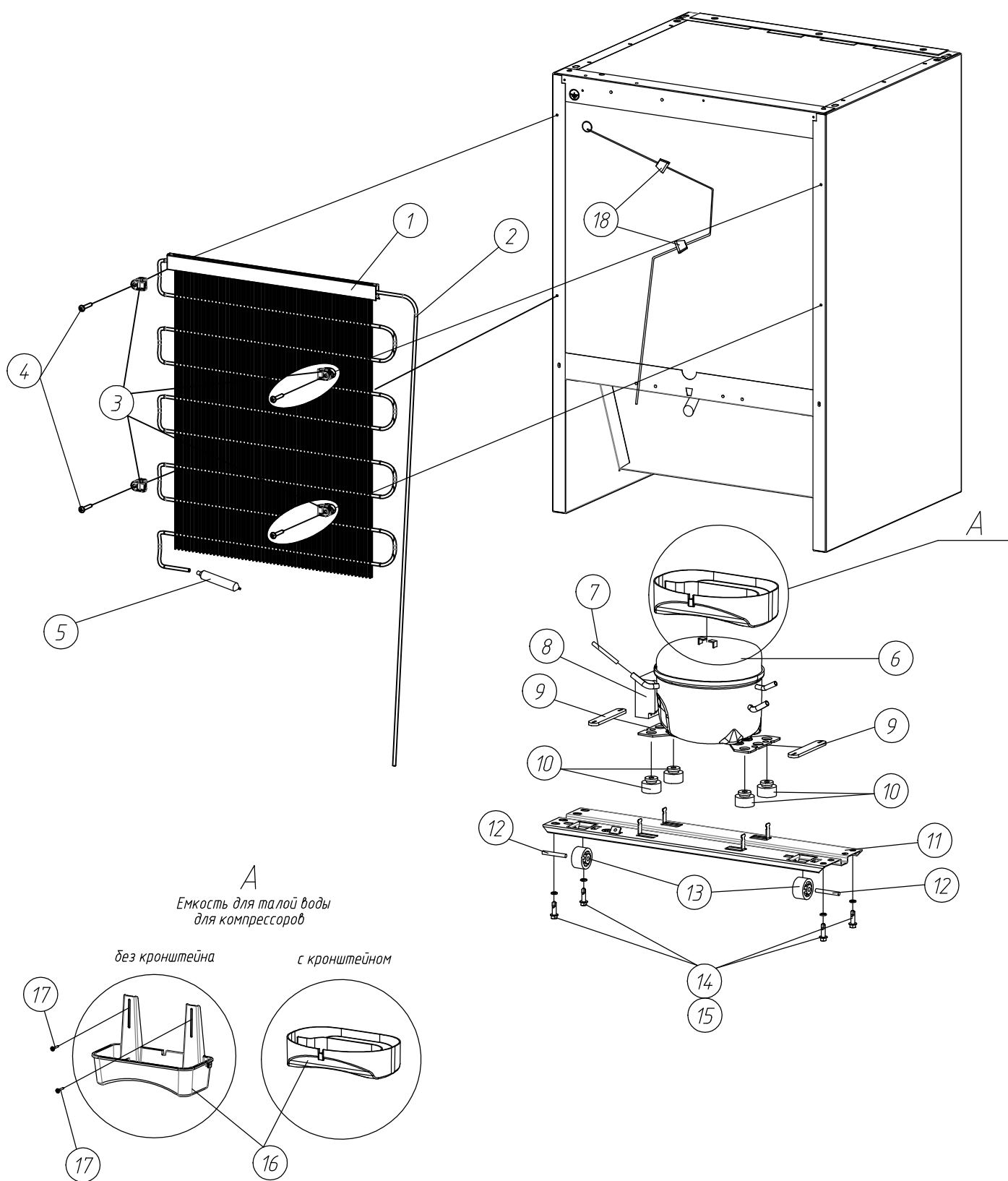
Рисунок 3 – Установка конденсатора и компрессора
