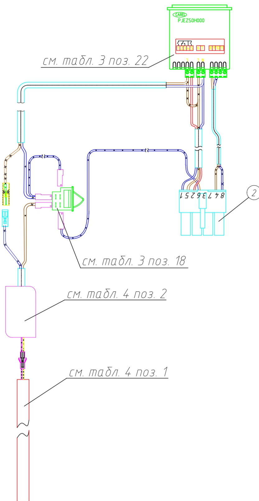
Рисунок 6а – Блок приборов (запеленная дверь, электронный блок) (остальное см. рисунок 6)
