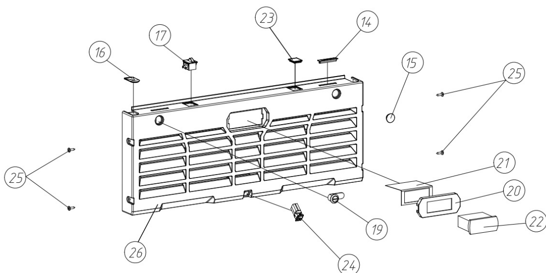
Рисунок 2а – Цокольная панель (стеклянная дверь+электронный блок+замок)
