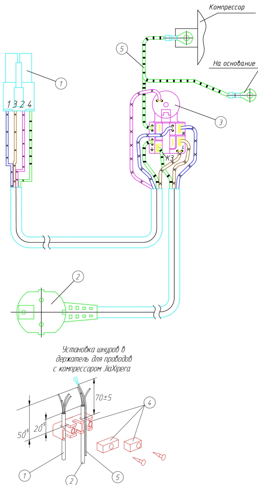
Рисунок 7 – Колодка компрессора в сборе
