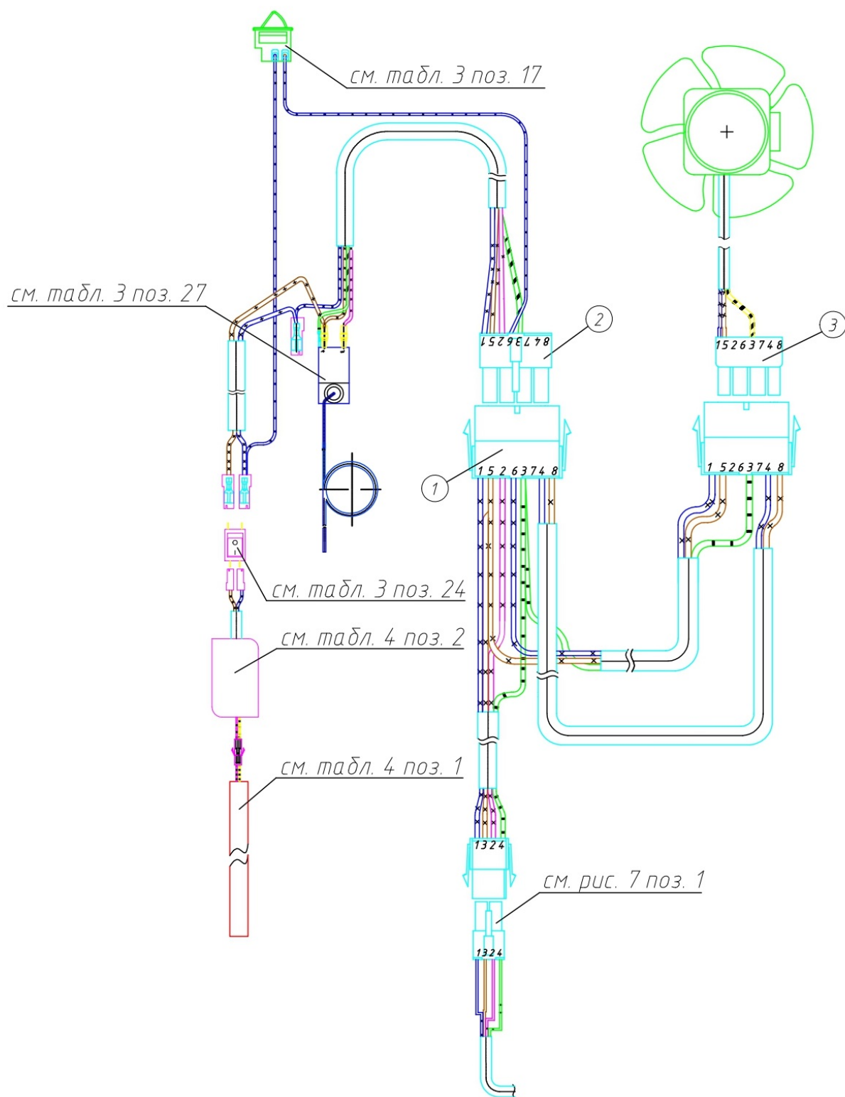
Рисунок 6б – Блок приборов (стеклянная дверь, механическое реле)
