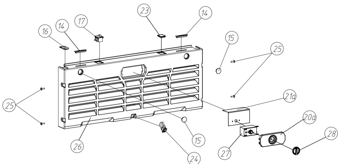
Рисунок 2в– Цокольная панель (стеклянная дверь+мех. реле)
