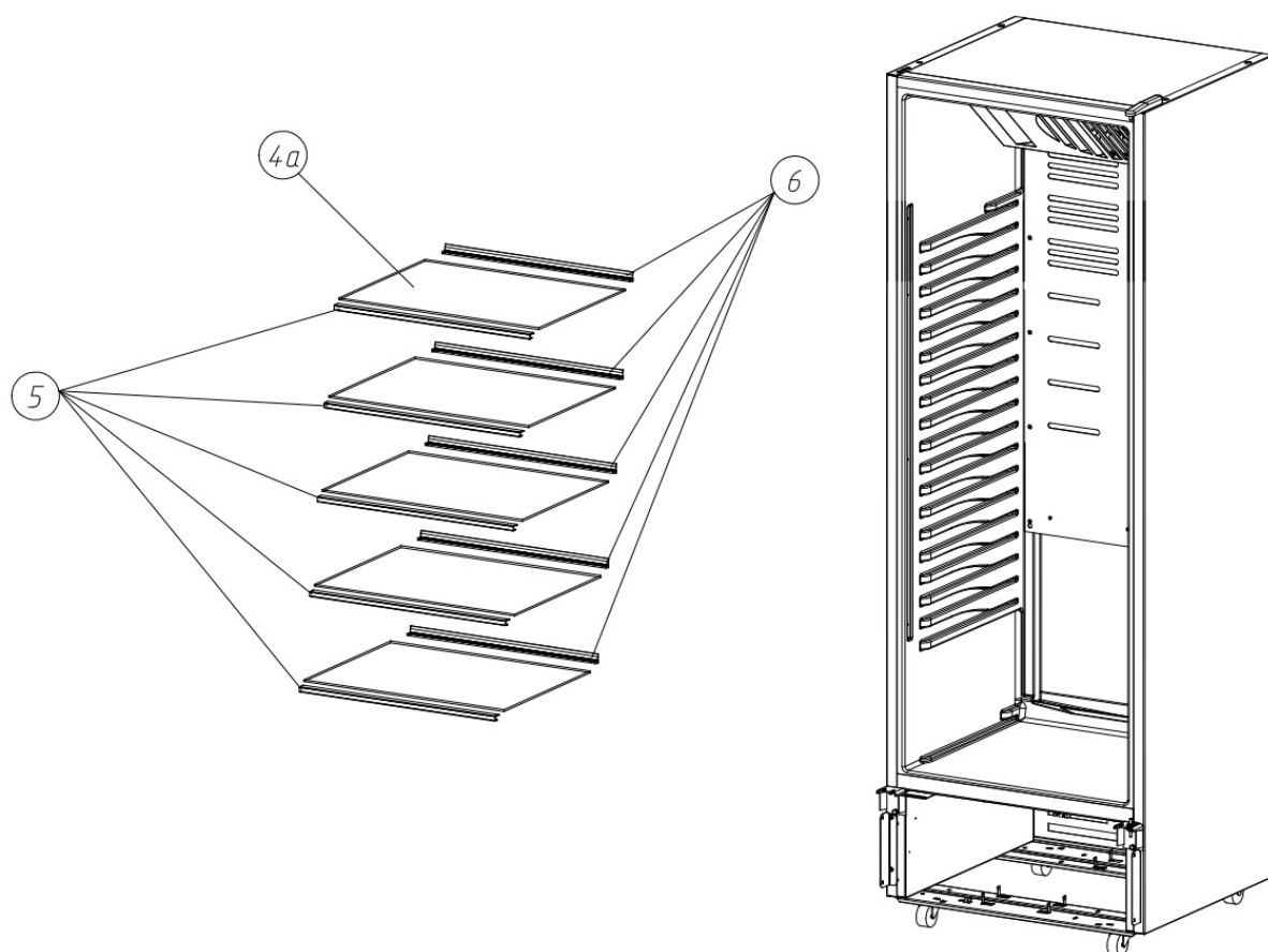
Рисунок 3а – Возможная комплектация
