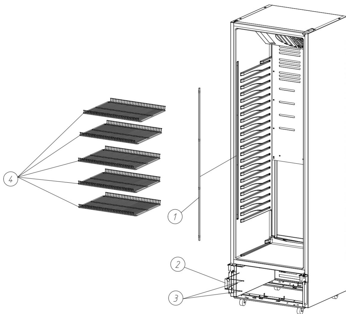
Рисунок 3 – Внутренние принадлежности шкафа
