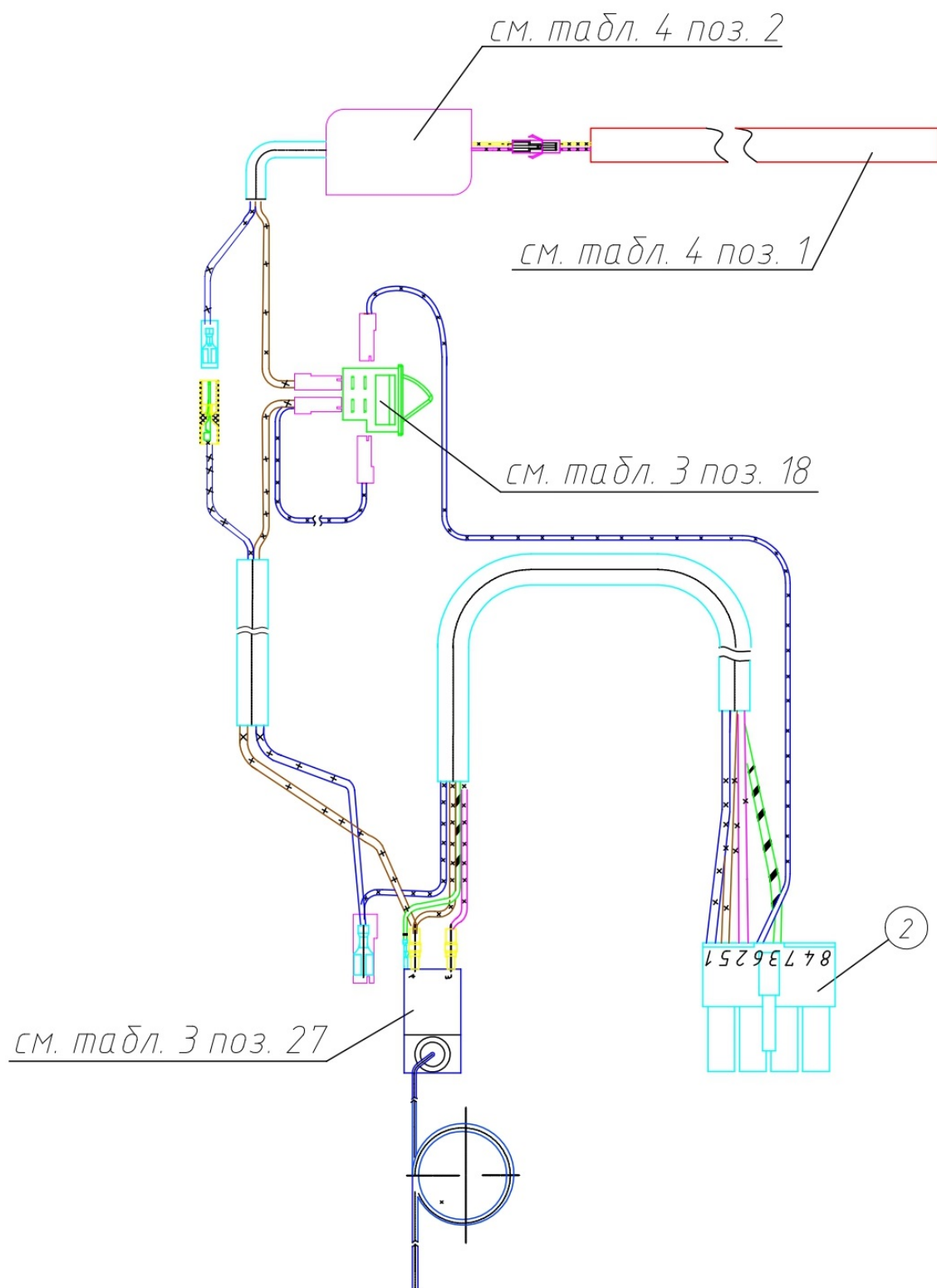
Рисунок 6в – Блок приборов (запеленная дверь, механическое реле) (остальное см. рисунок 6б)
