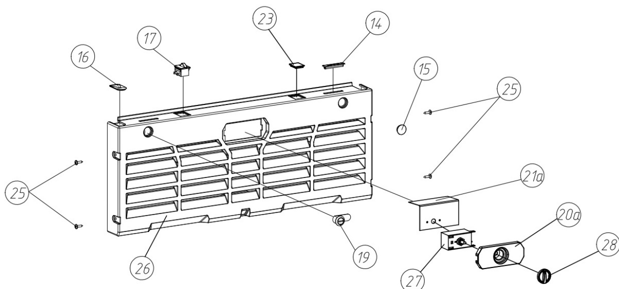
Рисунок 2г– Цокольная панель (запененная дверь+мех. реле+замок)
