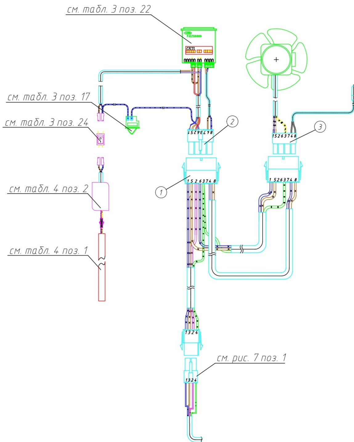
Рисунок 6 – Блок приборов (стеклянная дверь, электронный блок)
