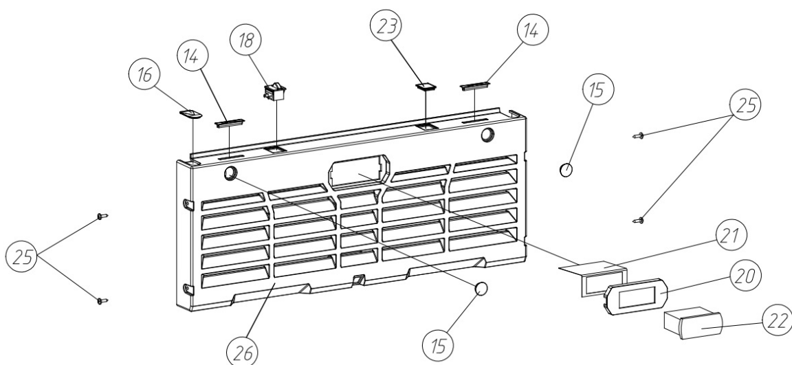
Рисунок 2б– Цокольная панель (запененная дверь+электронный блок)
