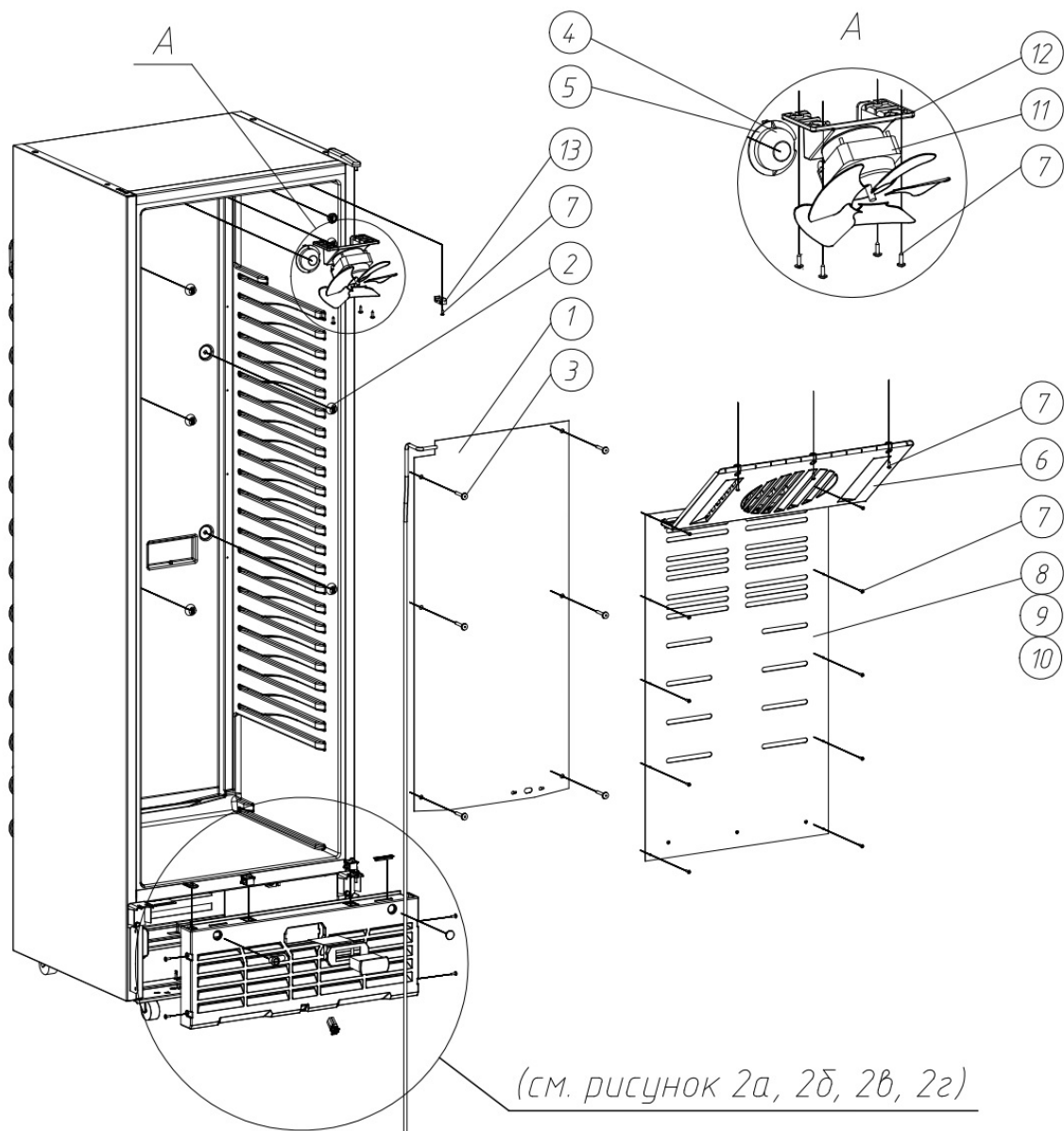
Рисунок 2 – Внутренние комплектующие шкафа
