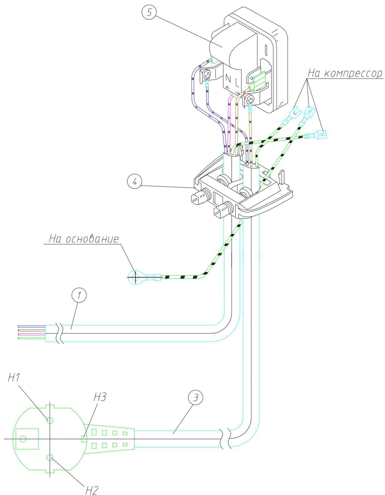
Рисунок 7а – Колодка компрессора в сборе (Secor NL10FT)
