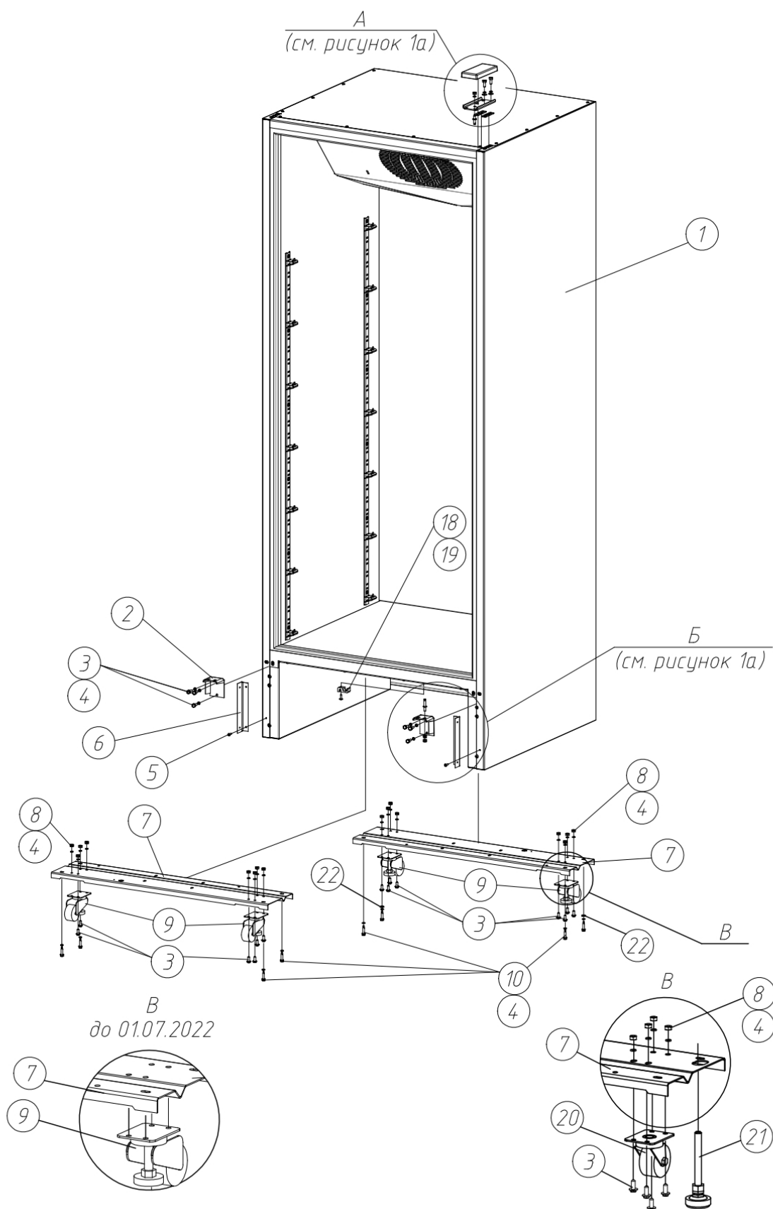
Рисунок 1 – Комплектующие шкафа
