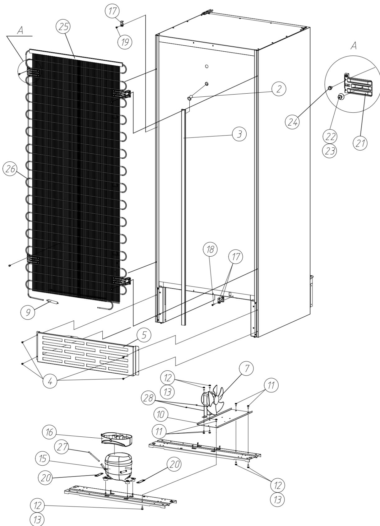
Рисунок 4а – Установка конденсатора и компрессора (для исполнений с навесным конденсатором)
