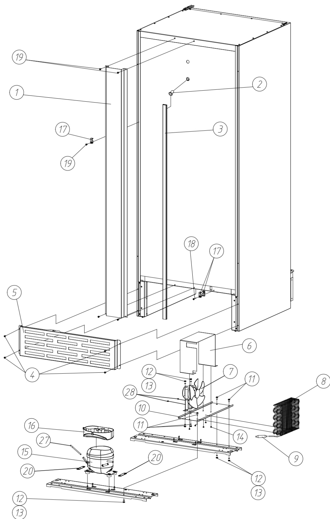
Рисунок 4 – Установка конденсатора и компрессора (для исполнений с обдувным конденсатором)
